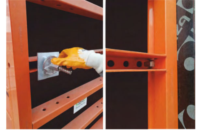
Rapido Köşe Birleştirme Detayı Rapido Corner Connection Detail
